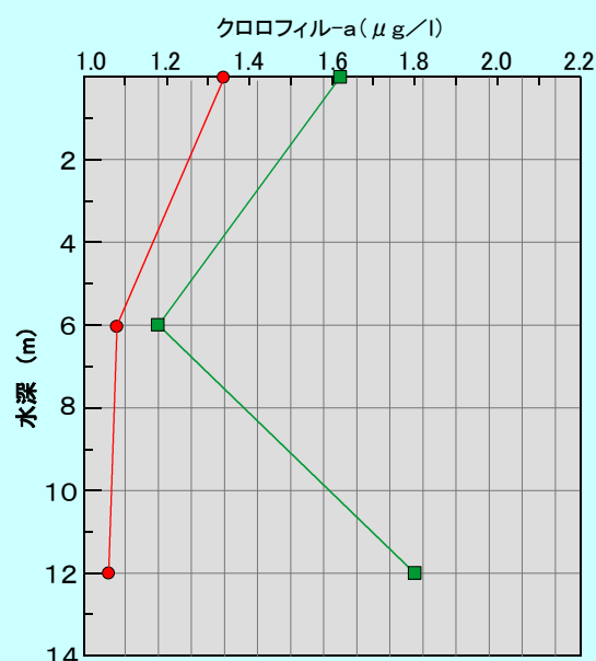
クロロフィルaの鉛直変化
