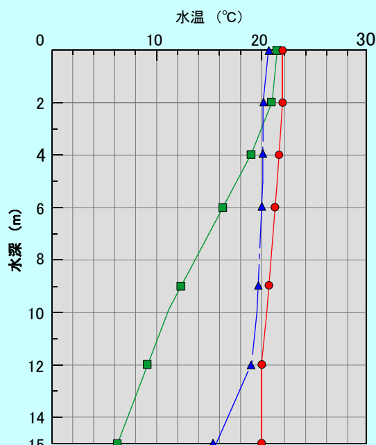
水温鉛直分布の変化
