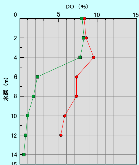
DO鉛直分布の変化
