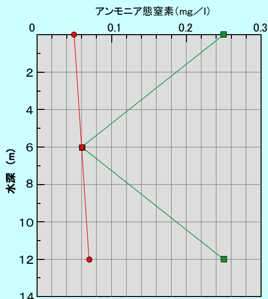
アンモニア態窒素の鉛直変化
